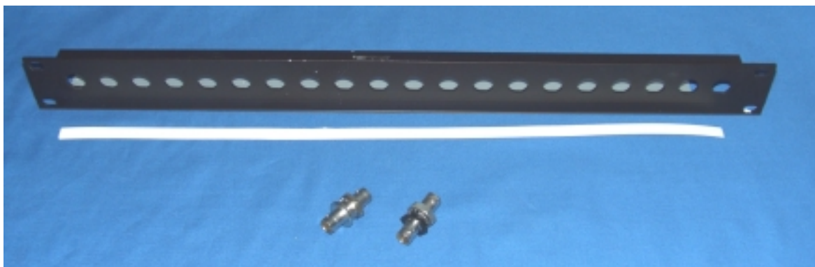
BNC-overgang hun/hun ujordet (plastisolasjon mot chassis) (DRS-1731-1U-BNC/75)
